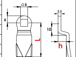
Mini Kilit Dilleri Mini Lock Cams
