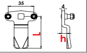
İspanyolet Diller Espagnolette Cams
